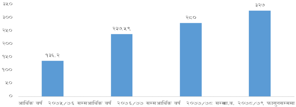
चार्ट ४.६ : प्रदेश नं १ को विद्युत उत्पादन क्षमता (वैकल्पिक ऊर्जा प्रवर्द्धन केन्द्रबाट उत्पादित विद्युत बाहेक)
